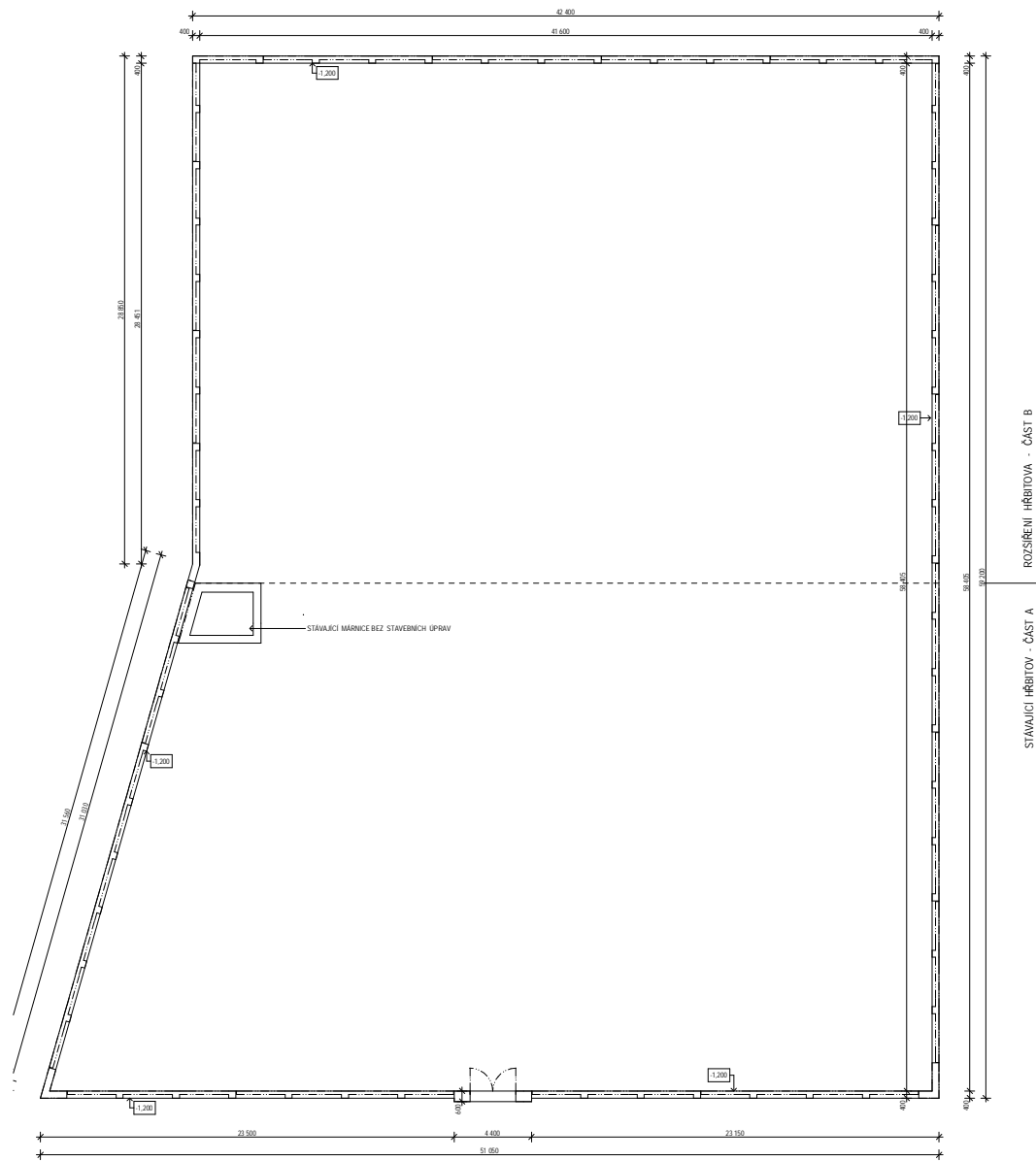
DETAIL ZÁKLADOVÉHO PASU M 1:50
